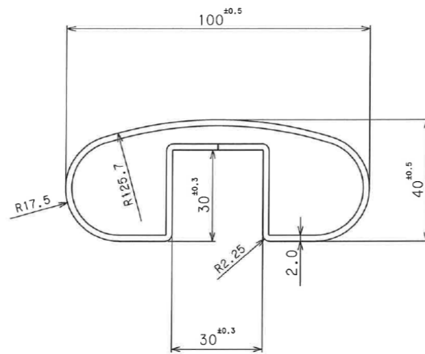
SUS304 異形楕円パイプ2.0×100×40
